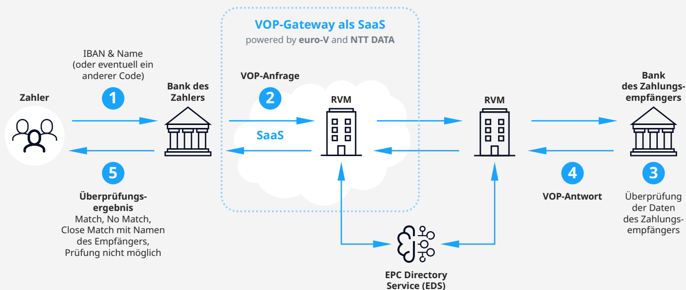
Ablauf einer VOP-Anfrage
